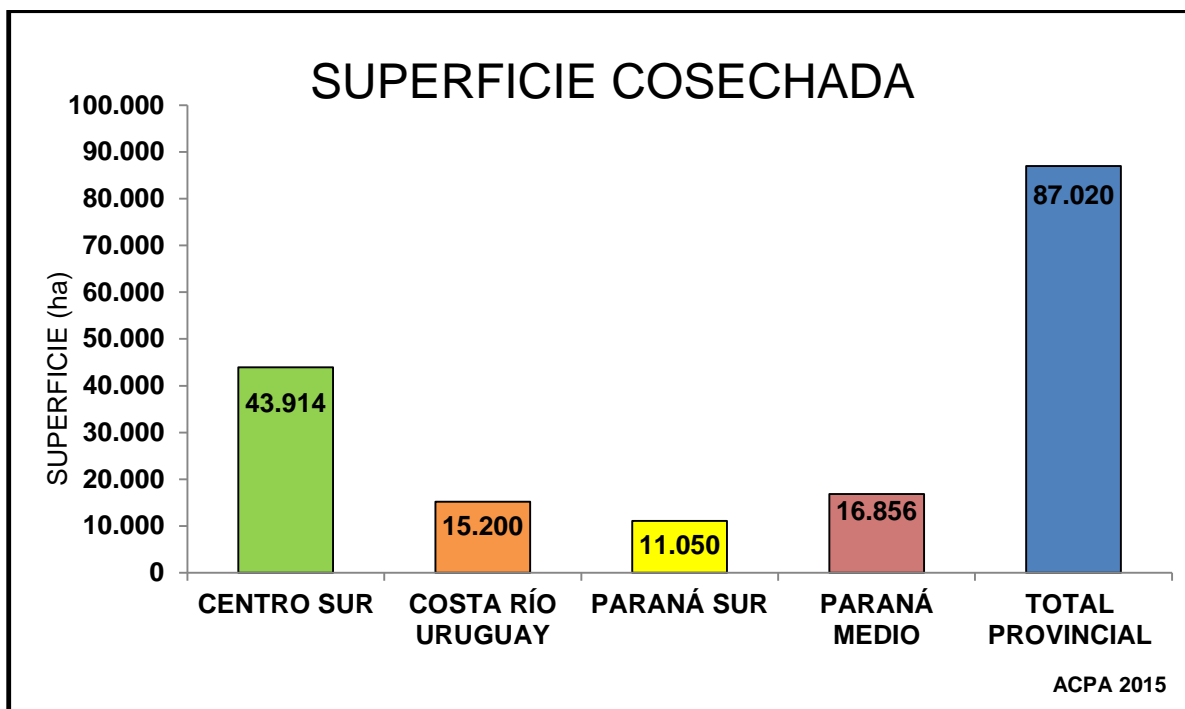
Gráfico N°1: Superficie cosechada por zona productiva.
