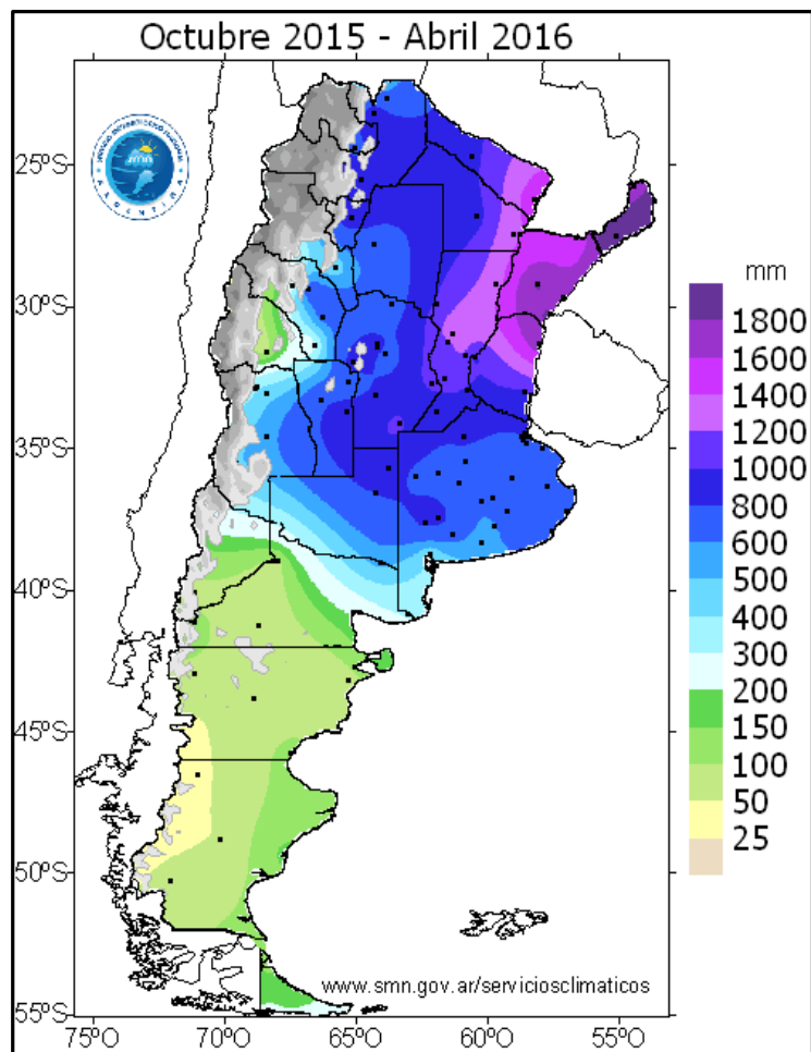
Precipitaciones acumuladas desde el mes de Octubre 2015 a Abril de 2016.
